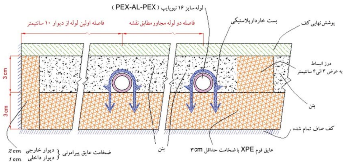
مقطع لایه بندی سیستم گرمایش از کف SGP
