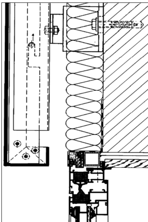
شکل پ-۱۰ مقطع عمودی اتصال پنجره به نما در صورت نصب به روش آویخته
