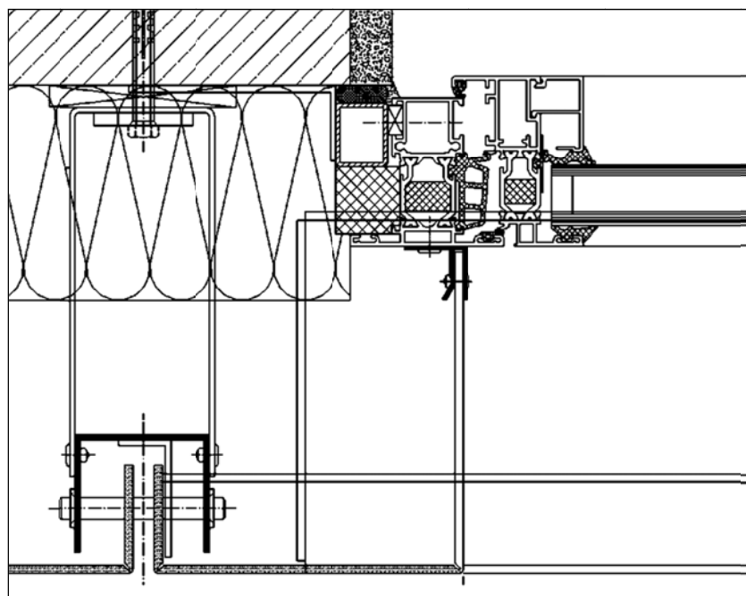
شکل پ-۱۱ مقطع افقی اتصال پنجره به نما در صورت نصب به روش آویخته
