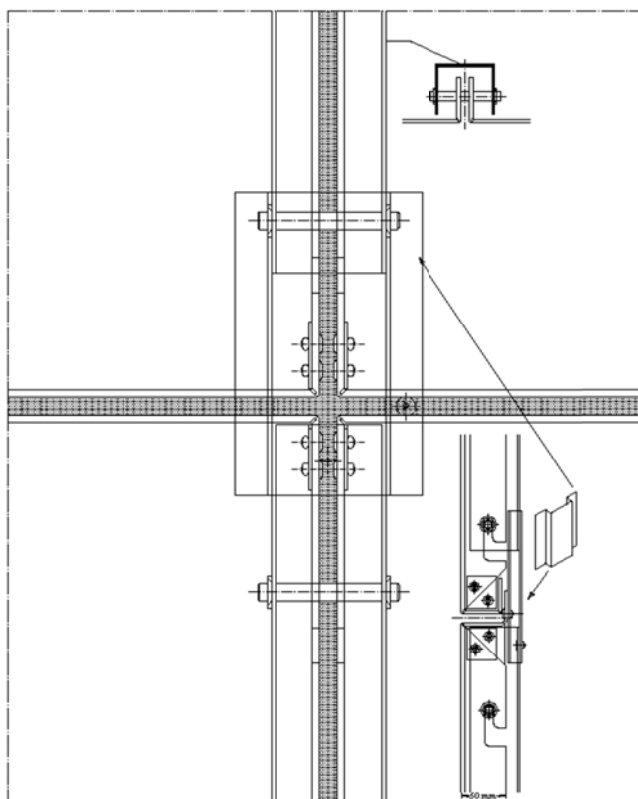
شکل پ-۸ نما و مقطع افقی وعمودی اتصال قطعات به قلاب در صورت نصب به روش آویخته
