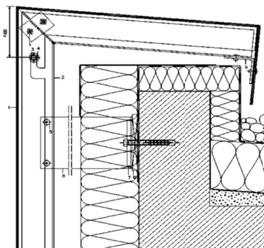
شکل پ-۱۴ مقطع عمودی نمونه اجرای پوشش روی جان پناه
