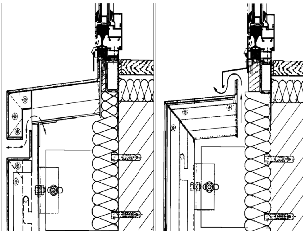
شکل پ-۹ مقطع عمودی روش های مختلف اتصال پنجره به نما و ایجاد جریان هوا در صورت نصب به روش آویخته
