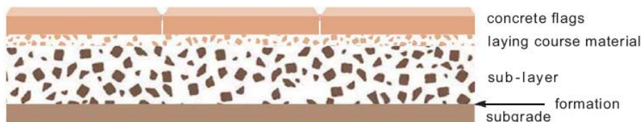
شکل ۱-۱- اجزای اصلی روسازی با سنگ‌فرش بتنی
