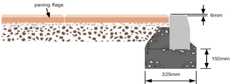
شکل ۱-۴- لبه‌گذاری با جدول بتنی پیش‌ساخته (مناسب برای عبور خودرو از روی آن)
