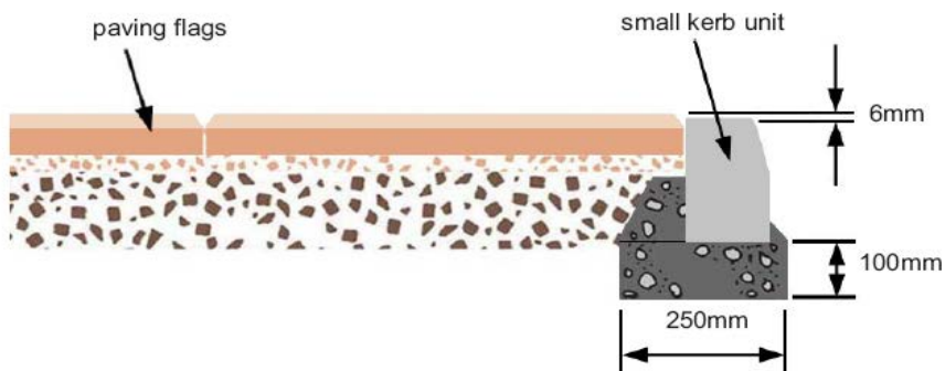
شکل ۱-۳- لبه‌گذاری با جدول‌های کوچک (مناسب برای عبور خودرو از روی آن)
