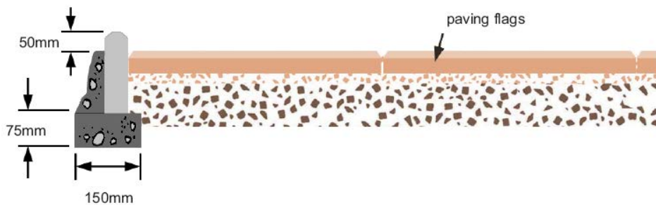
شکل ۱-۲- لبه‌گذاری پیش‌ساخته بتنی (نامناسب برای عبور خودرو از روی آن)
